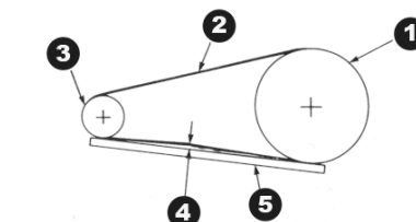
Figure 4: Réglage de la courroie de ventilateur
