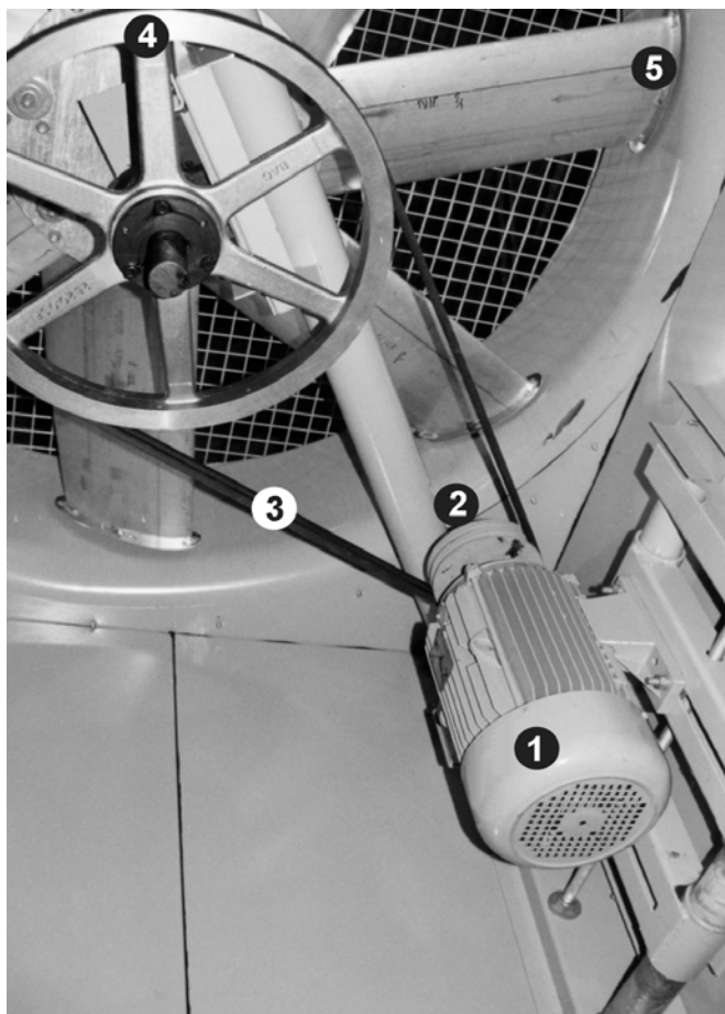
Figure 6: Système d'entraînement
