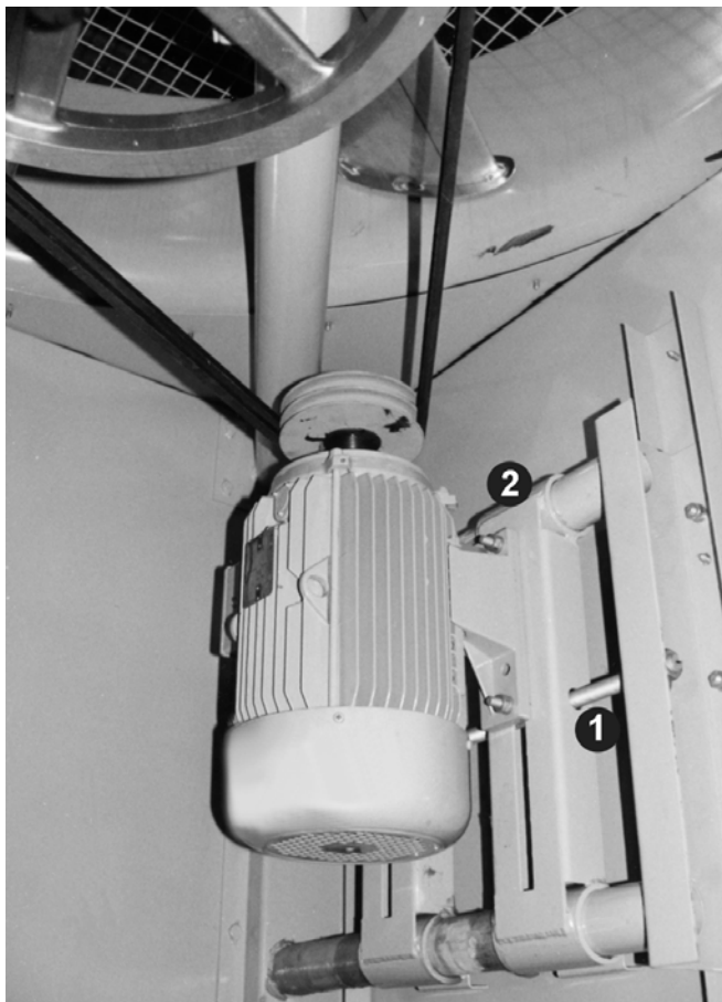
Figure 14: Chaise moteur réglable
