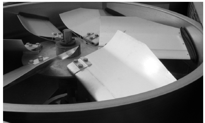
Figure 12: Ventilateur axial
