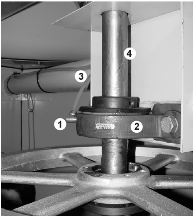
Figure 11: Emplacement des paliers d'arbres de ventilateurs et des graisseurs
