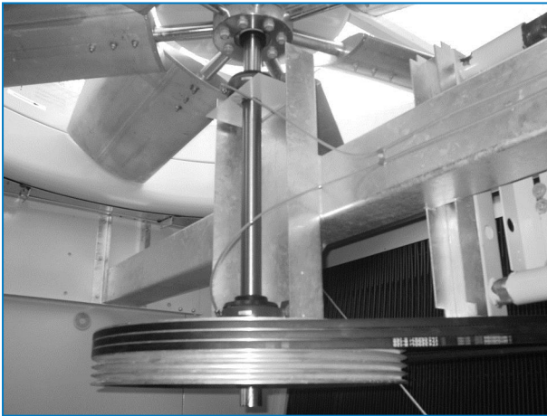
Fan shaft
